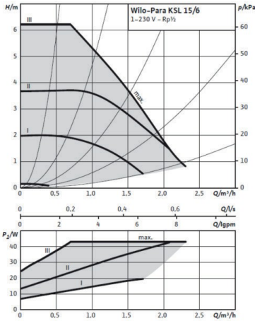
Üç Kademeli Çalışma Eğrisi (Eğri 3)
