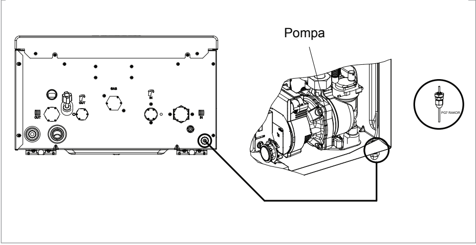
Şekil 17. Dış hava sensörü ve oda termostatu kabloları geçiş rakoru ve konumu
