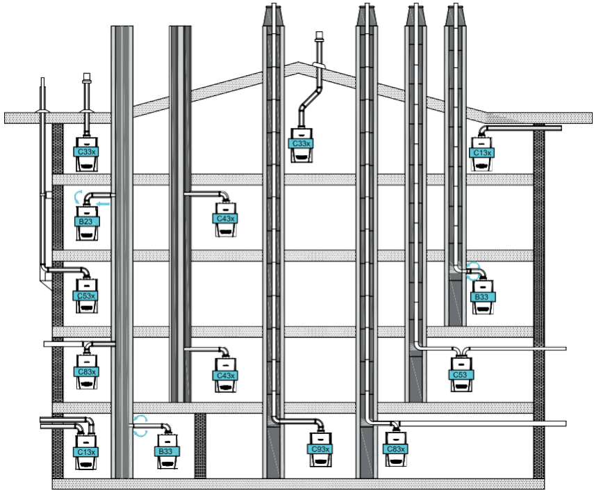
Şekil 23. Baca uygulamaları
