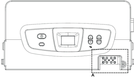
Şekil 17. Dış hava sensörü ve oda termostatu kabloları geçiş rakoru ve konumu
