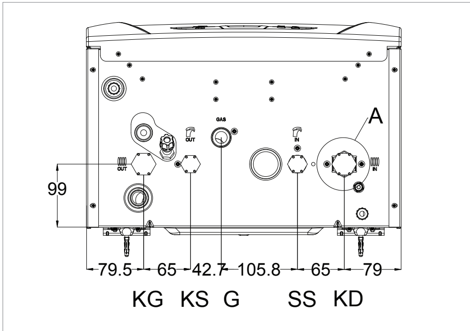
Şekil 15. Su bağlantıları
