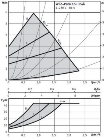
Üç Kademeli Çalışma Eğrisi (Eğri 3)
