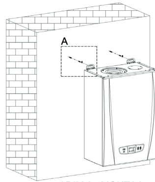
ADIM 2 - MONTAJ
