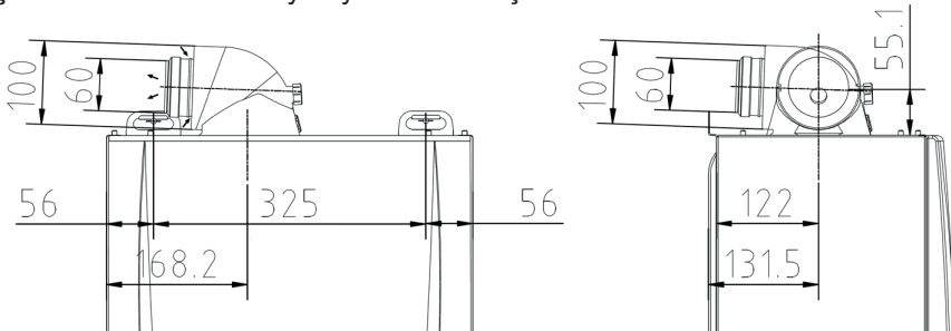
Şekil 26. Ø60/100 mm yatay baca seti ölçüler
