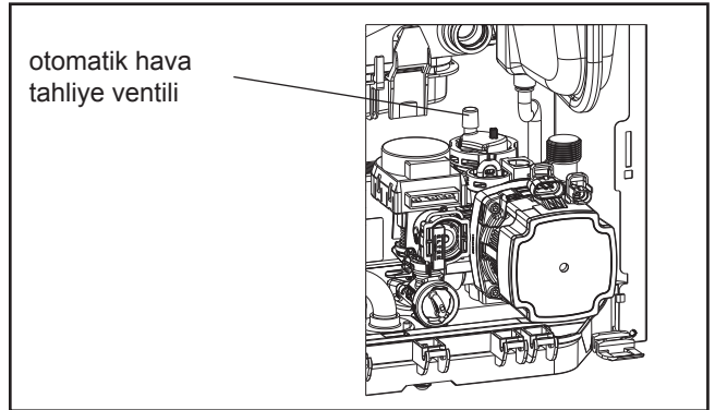
Resim: Isıtma devresi pompasında bulunan otomatik hava tahliye ventilii
