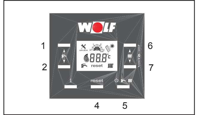
Resim: Kontrol paneli tuşları
