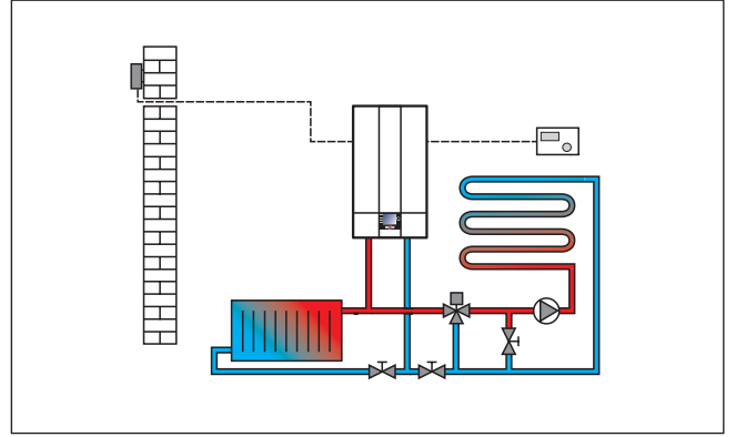
Resim: Yerden ısıtma sistemi
