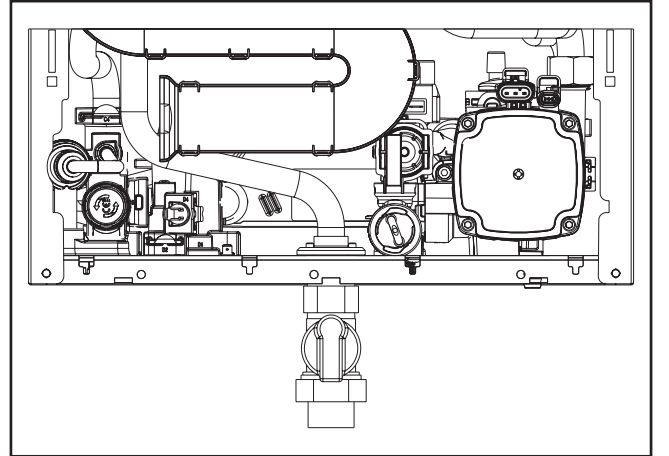
Resim: Gaz bağlantısı montajı
