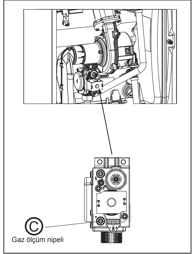
Resim: Gaz bağlantı basıncının değiştirilmesi
