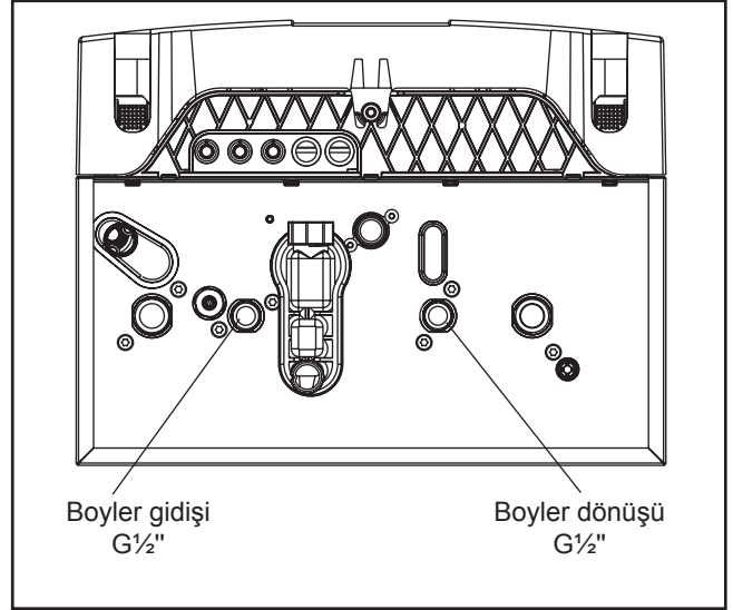
Resim: Boiler gidiş / dönüş bağlantısı
